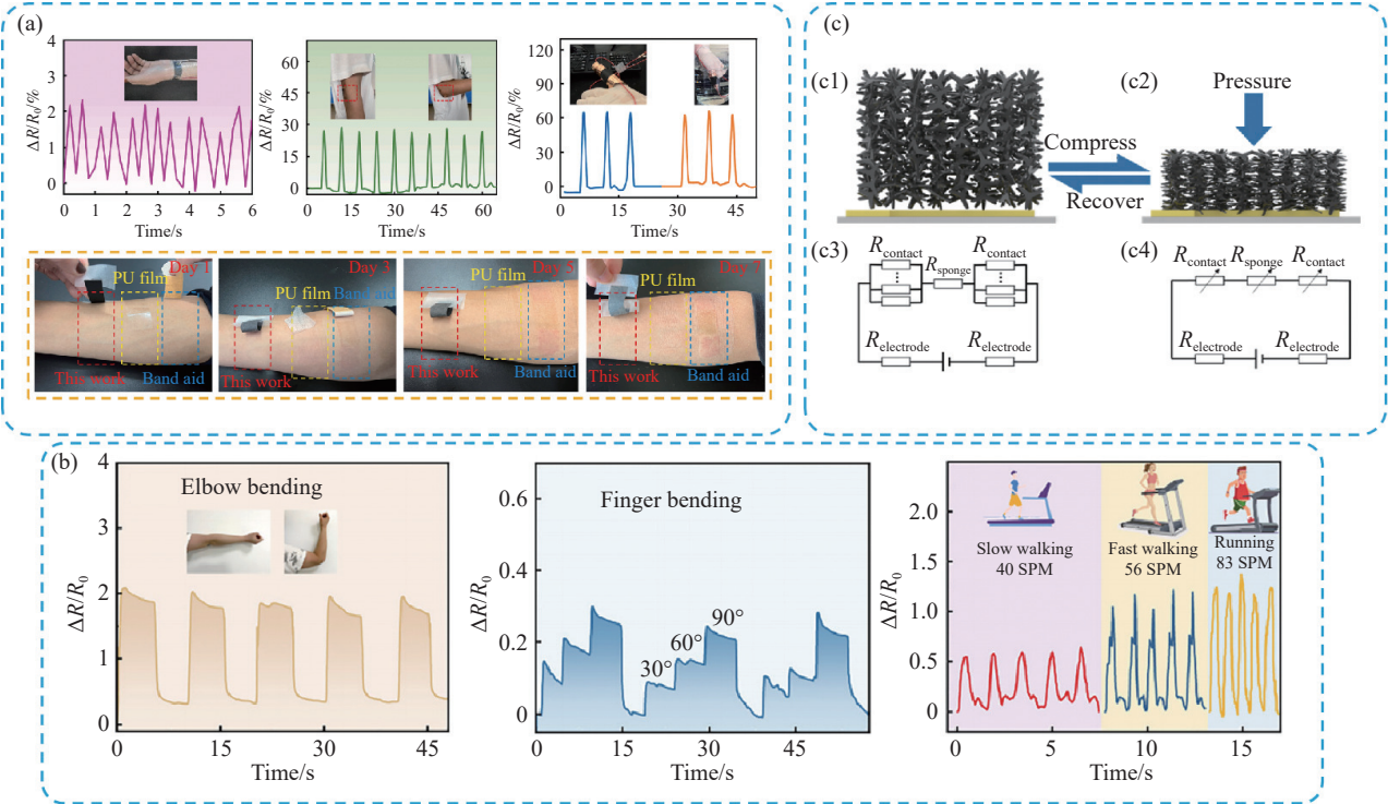
图3 以纤维制品为基体的MXene传感器用于动作监测：(a) 纸基MXene传感器运动监测及透气性比较测试；(b) 纺织品基MXene传感器监测动作；(c) 传感器工作原理示意图 [50-52]
