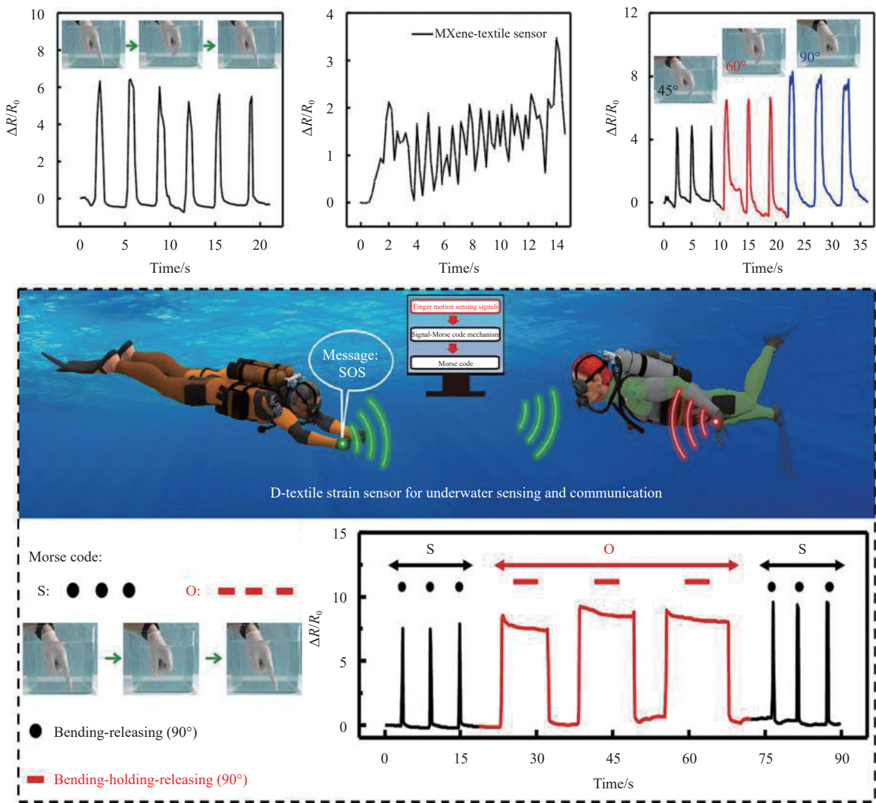
图7 具有超疏水涂层的MXene 纺织品用于水下运动监测 [81]
