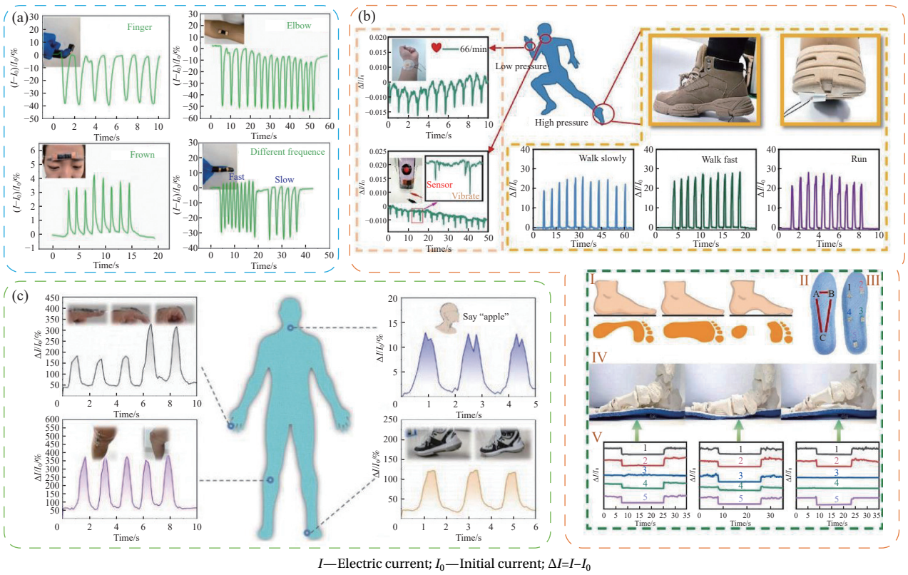
图4 以凝胶为基体的MXene传感器用于动作监测: (a) MXene复合明胶(MCG)传感器监测手指、肘部运动; (b) 海藻酸钠/MXene/聚二甲甲基硅氧烷(SA/MXene/PDMS)气凝胶监测足部运动和步态; (c) MXene/Wood水凝胶监测手指、膝盖运动 [59-61]
