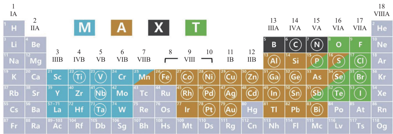
图1 MAX 和 MXene 相关元素 [37]
