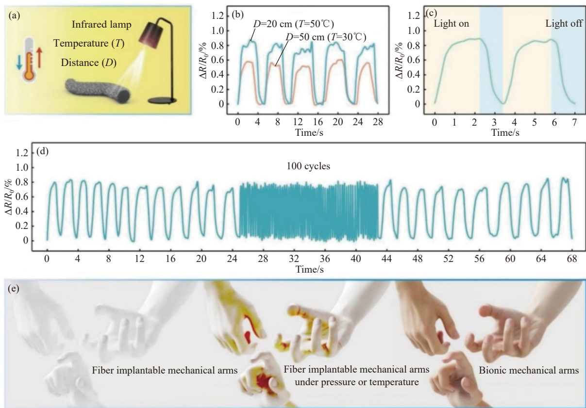
图 6 (a) 红外灯照射 PEDOT:PSS 基纤维图示；(b) 纤维在不同距离下的电阻变化 ( \Delta R/R_0 )；(c) 纤维电阻变化的响应时间；(d) 纤维在相同距离 ( D=20\text{ cm} 、 T=50^\circ\text{C} ) 红外灯的 100 次周期性开/关下的传感性能；(e) 纤维用于仿生手臂感知压力和温度的概念应用 [49]
