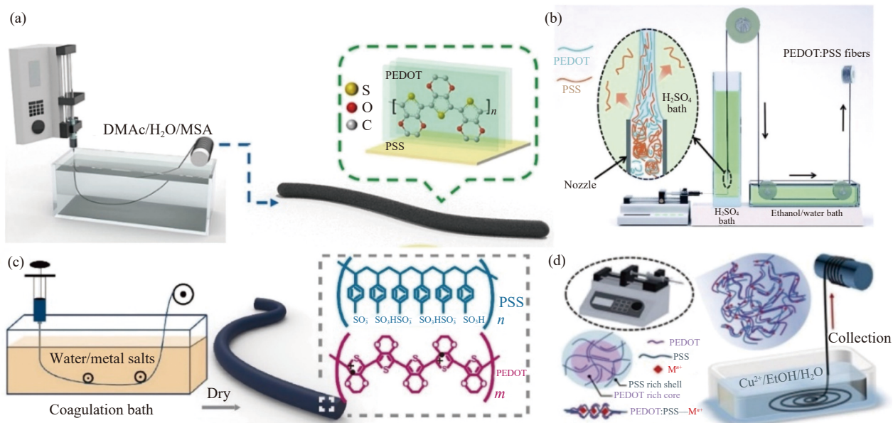
图3 不同组分凝固浴的调控: (a) N, N-二甲基乙酰胺 (DMAc)/ \text{H}_2\text{O} /甲基磺酸 (MSA) [44] ; (b) \text{H}_2\text{SO}_4 [42] ; (c) \text{H}_2\text{O} - \text{Fe}^{3+} [43] ; (d) EtOH- \text{H}_2\text{O} - \text{Cu}^{2+} [40]
