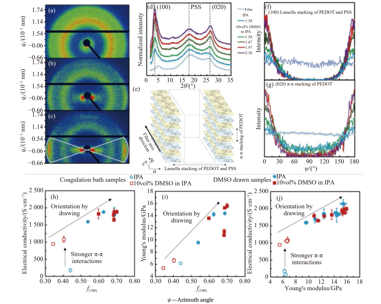
图 5 拉伸对湿纺 PEDOT:PSS 纤维性能的影响 [48] : (a) PEDOT:PSS 膜; (b) 对 PEDOT:PSS 纤维进行拉伸; (c) 进一步拉伸的 WAXS 分析; (d) 归一化强度(相对于 PSS 宽峰)与 2\theta 的关系; (e) PEDOT:PSS 晶体结构的示意图; (100) 反射(f) 和 (020) 反射(g) 的方位角的函数; 电导率(h)、杨氏模量(i)与聚合物链取向的关系; (j) 电导率与杨氏模量的关系
